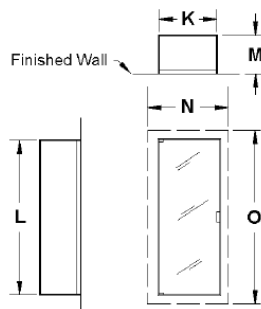
TRIMLESS
